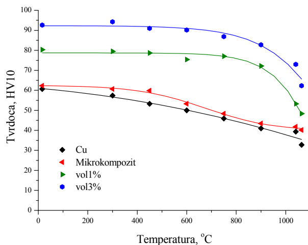
Slika 1. Promena tvrdoće HV10 bakra i različitih kompozita u funkciji temperature Figure 1. Dependence of hardness HV10 of copper and different composites from temperature
