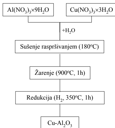
Slika 3 Šematski prikaz termohemijske sinteze Cu- \text{Al}_2\text{O}_3 nanokompozitnih materijala Figure 3. Scheme of thermochemical synthesis of Cu- \text{Al}_2\text{O}_3 nanocomposite materials
